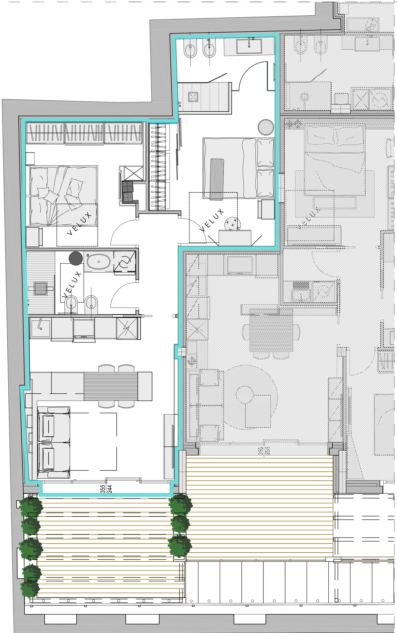
UNITA' IMMOBILIARE N.3 - PIANO TERRA SCALA 1:50
