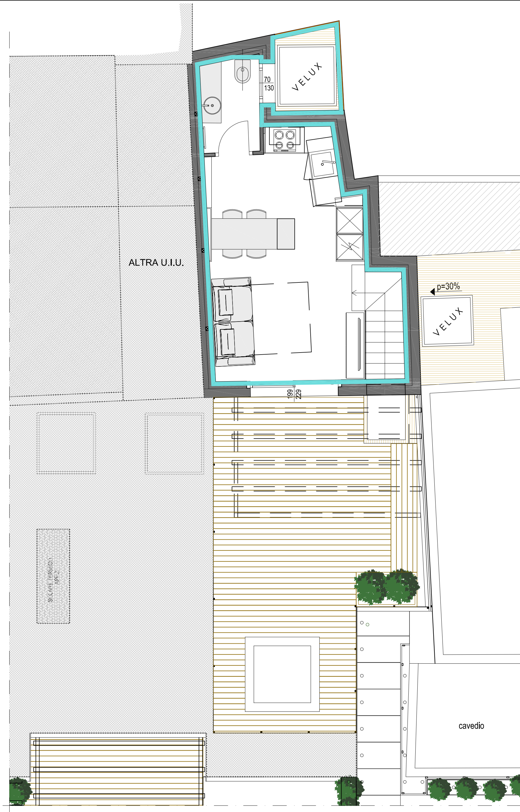
UNITA' IMMOBILIARE N.1 - PIANO PRIMO SCALA 1:50
